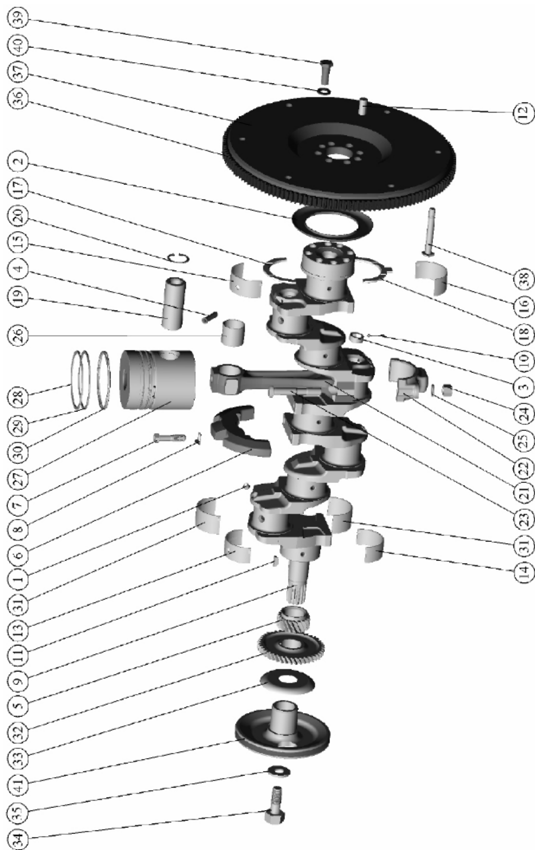
Рис. 10.1. Поршни и шатуны. Вал коленчатый и маховик
