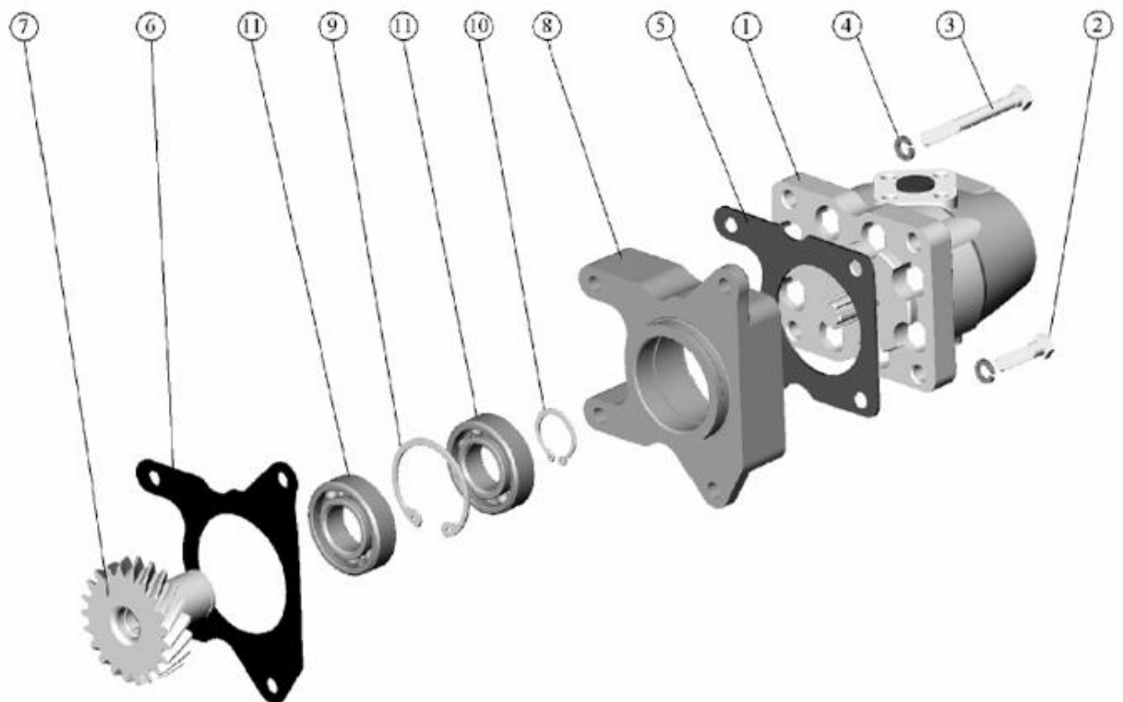
Рис. 10.1. Установка насоса рулевого управления
