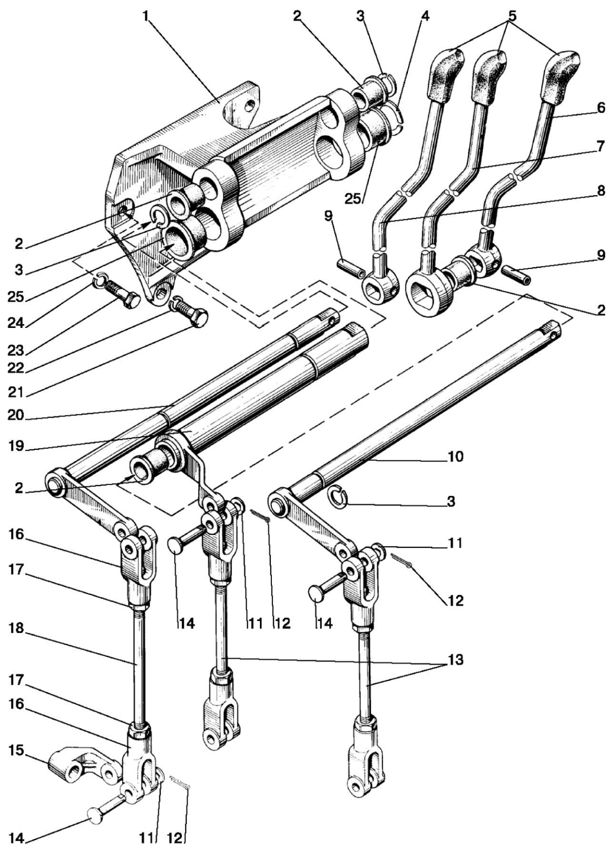
Рис. 10.1. Механизм задней навески
