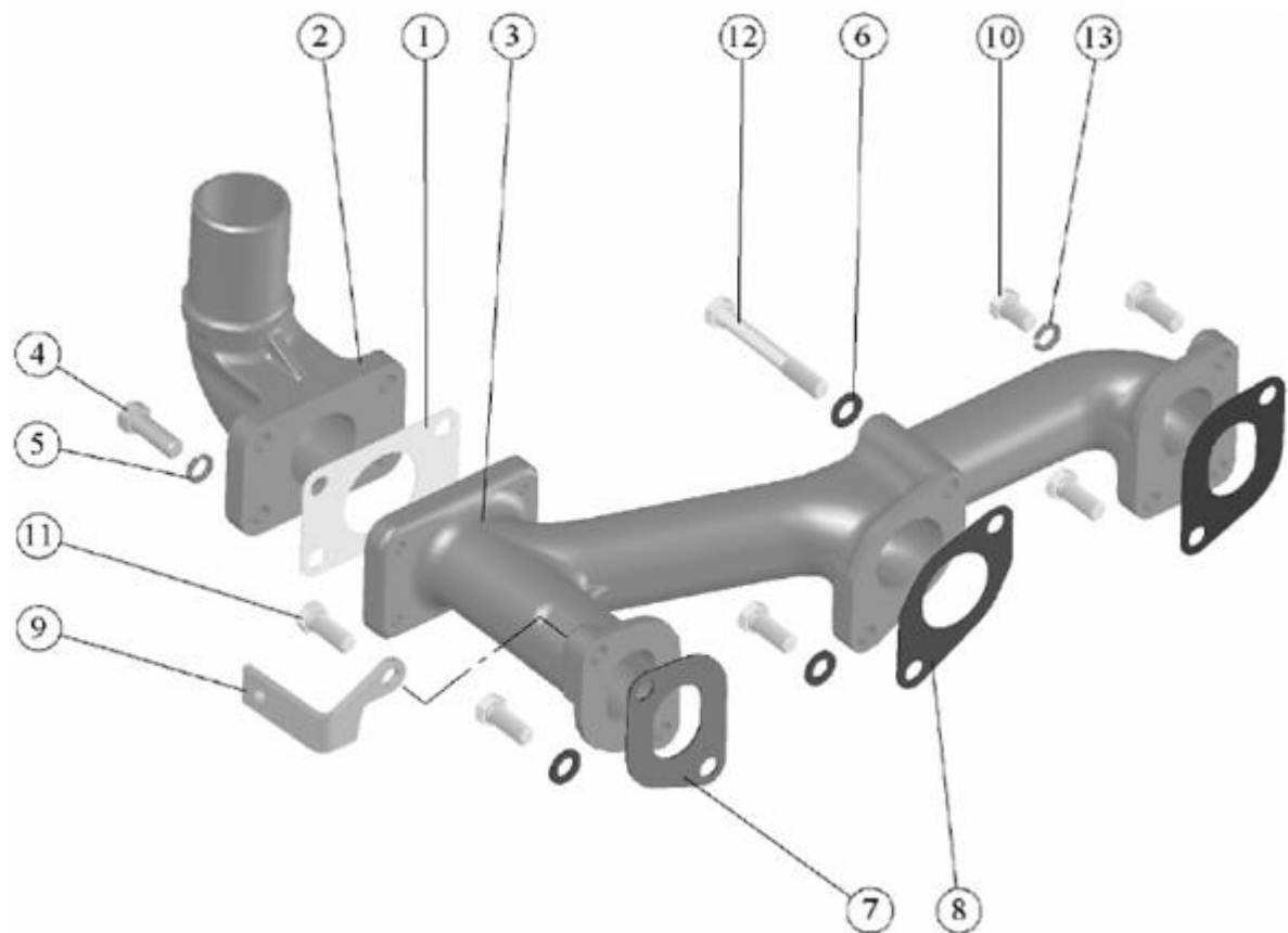
Рис. 10.1. Газопровод дизеля
