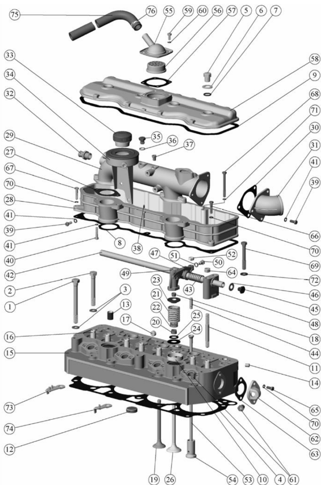
Рис. 10.1. Головка цилиндров. Клапаны и толкатели клапанов
