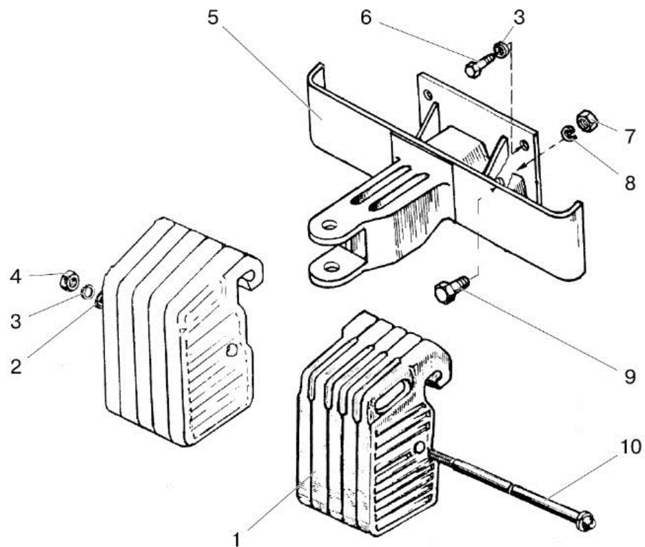
Рис. 10.1. Балласт передний
