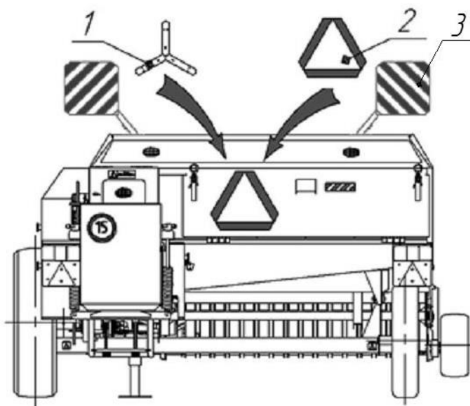
1 - кронштейн; 2 - знак «Тихоходное транспортное средство»; 3 - кронштейн с знаком «Крупногабаритный груз»
