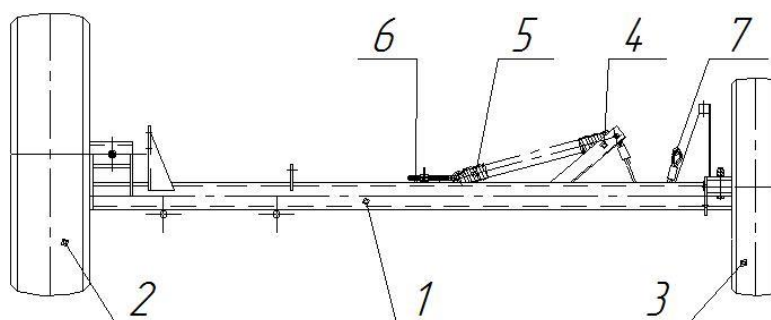
1 - основание; 2 - колесо; 3 - колесо; 4 - качалка; 5 - пружина; 6 - винт; 7 - трос.
