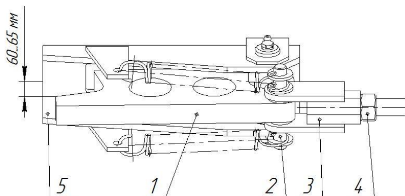
1 – упор; 2 – ось; 3 – вилка; 4 – гайка; 5 – кронштейн
