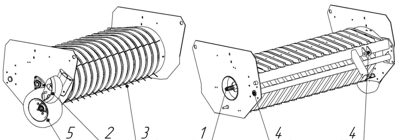
1 - вал приводной; 2 - дорожка; 3 - зубья пружинные; 4 - палец; 5 - колесо опорное.
